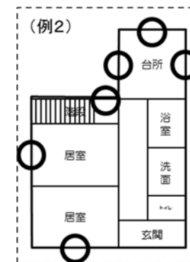
例2：断熱仕様が記載されている図書がない場合、連続する壁の面ごとに検査箇所を1カ所以上抽出して目視確認。
